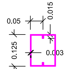
DETALLE PERFILERIA PARA NOVALOSA 2G 125x50x15x3mm Esc. 1 = 5
