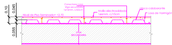
Detalle de conectores sobre vigas secundarias
