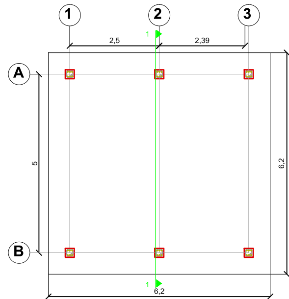
PLANTA DE LOSA DE CIMENTACIÓN Esc 1=50
