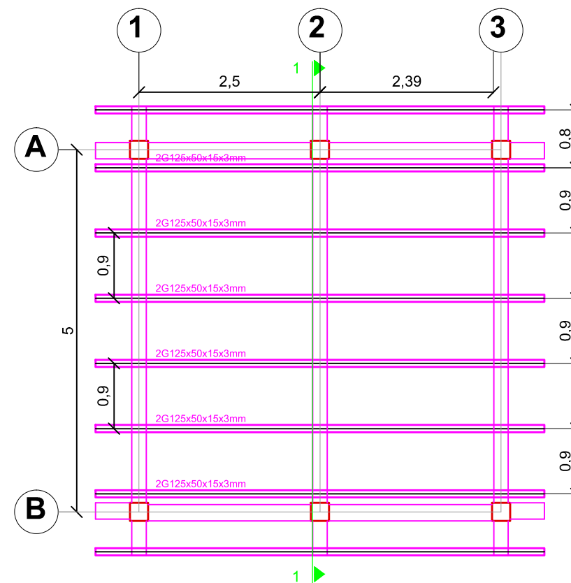
PLANTA DE NOVALOSA Esc. 1=50
