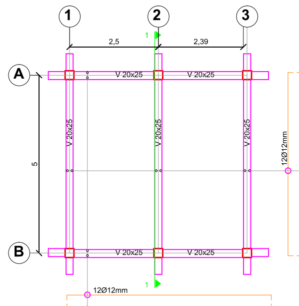
PLANTA DE VIGAS SUPERIORES Esc. 1=50
