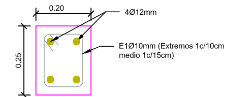
DETALLE VIGAS V(20x25cm) Esc. 1=5
