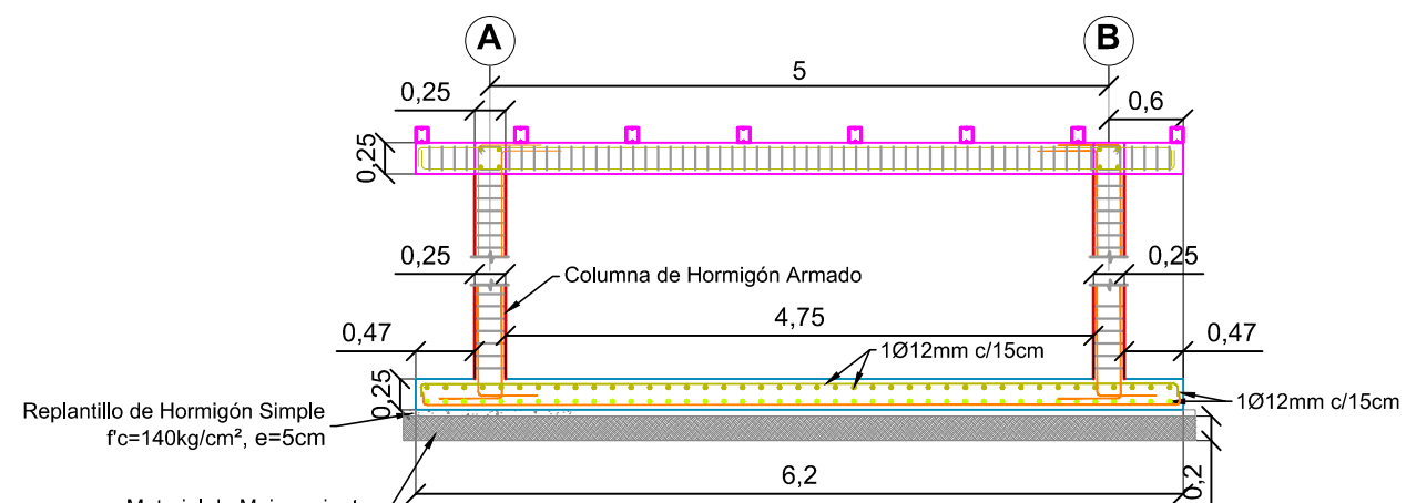
DISTRIBUCIÓN HIERROS CORTE 1 - 1 Esc 1=50
