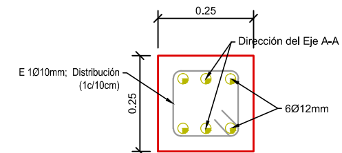
DETALLE COLUMNAS C1 (25x25) Esc. 1=5
