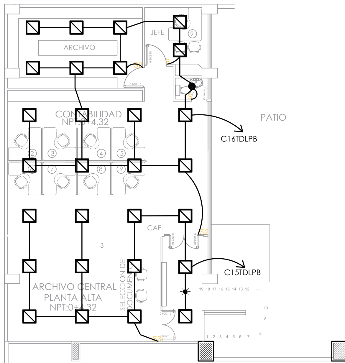
MEZZANINE: ARCHIVO CENTRAL / CONTABILIDAD NPT:0+4.32 ESCALA 1:100
