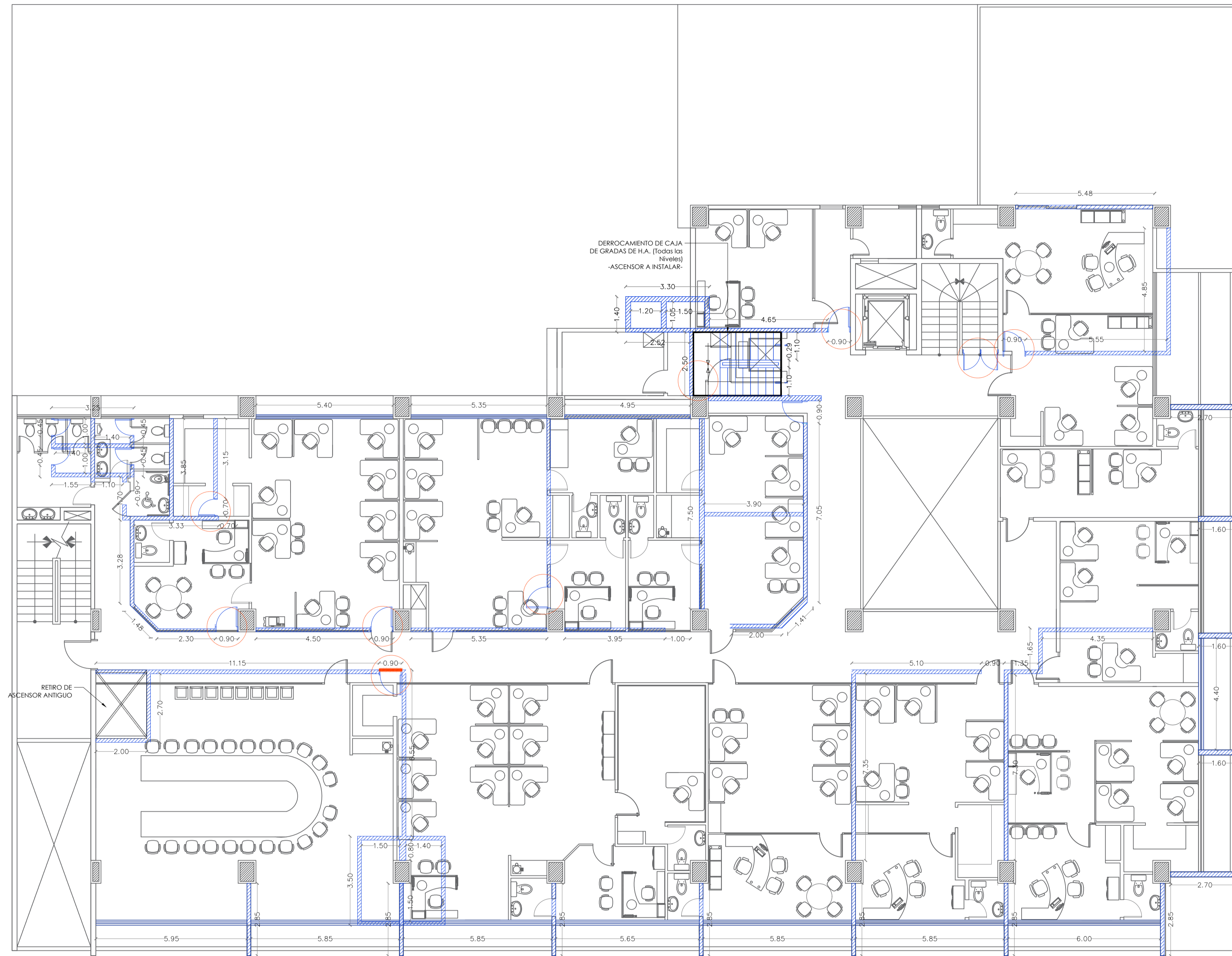
4° PLANTA ALTA N+11.68 ESCALA 1:100
