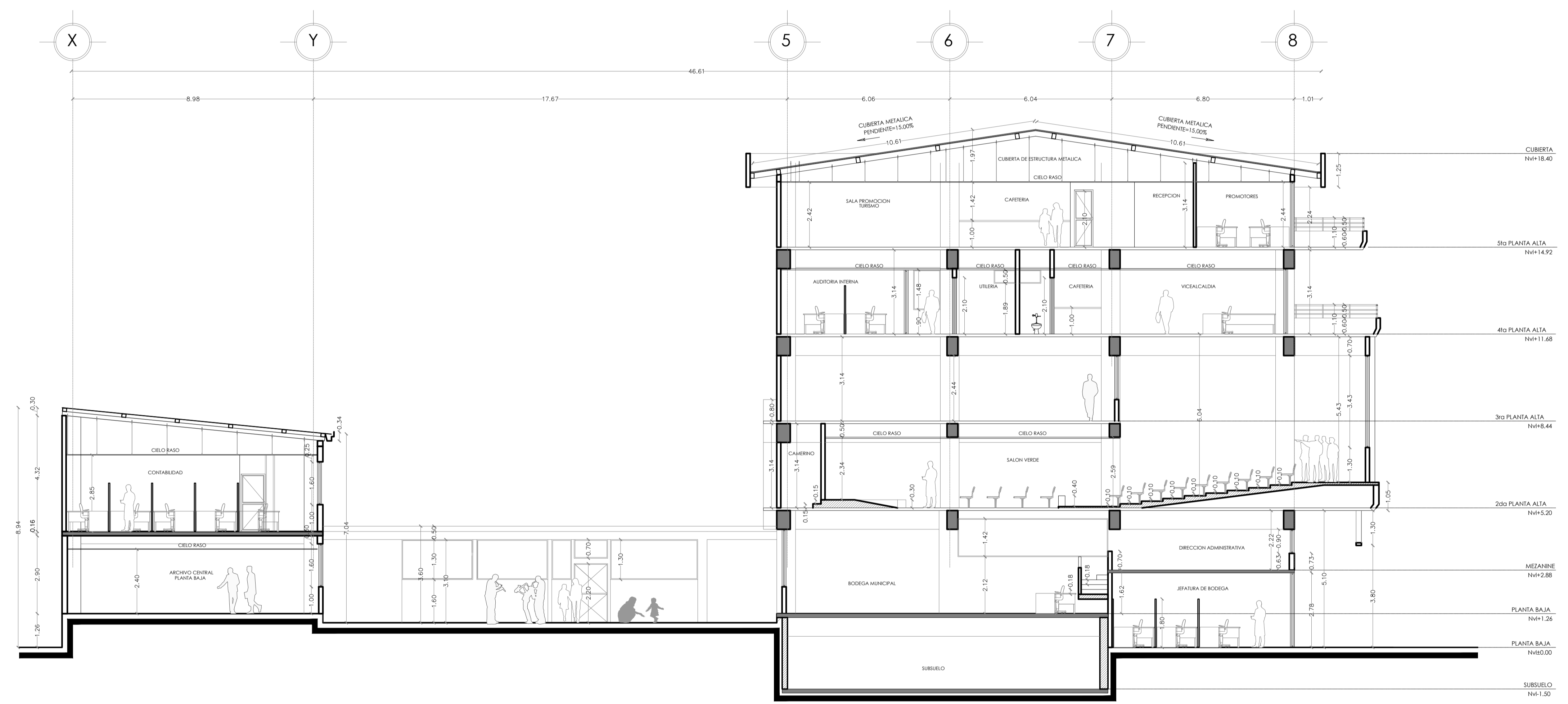
SECCION C-C ESCALA 1:100
