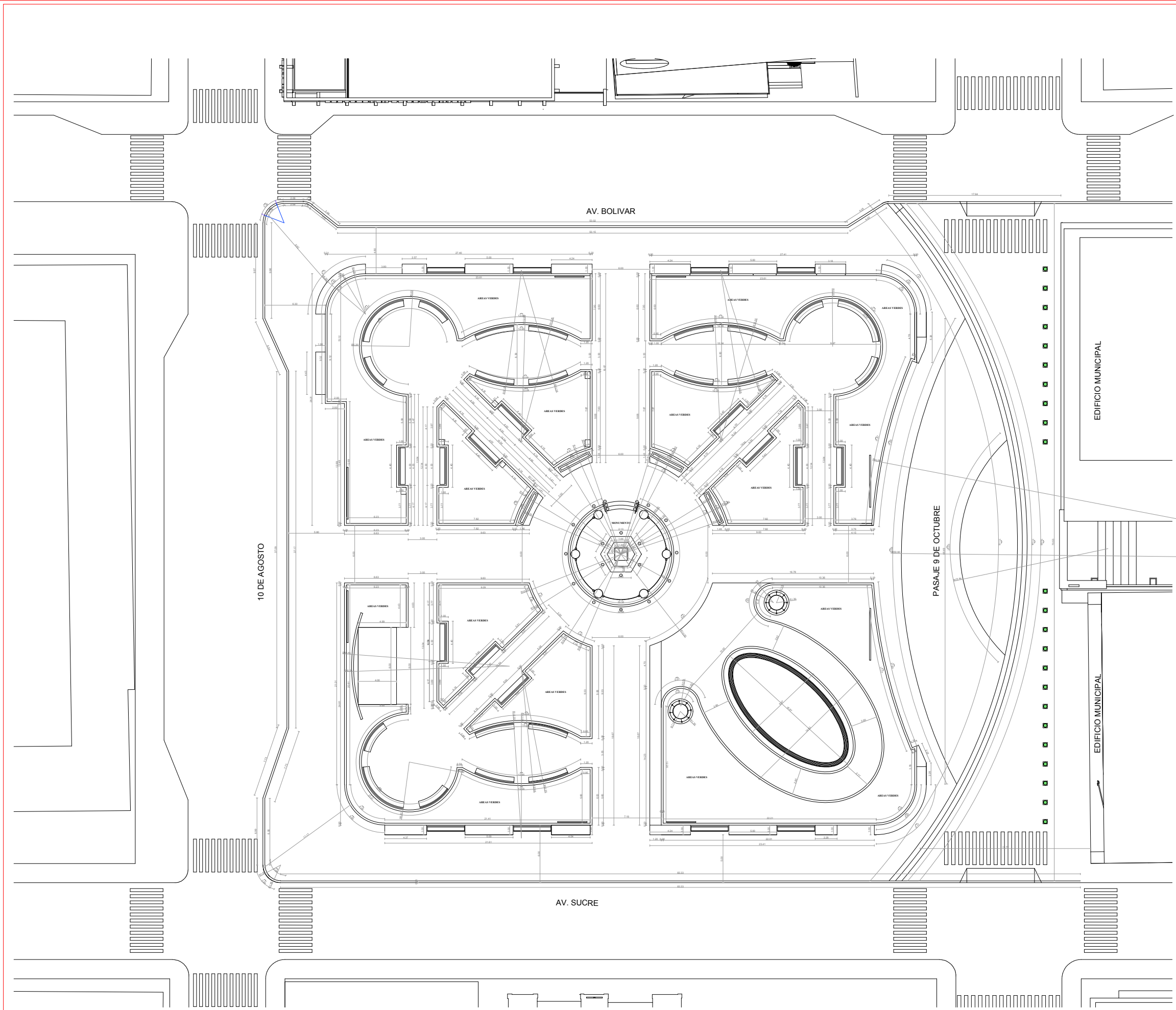
TRAZADO Y REPLANTEO ESCALA 1: 200
